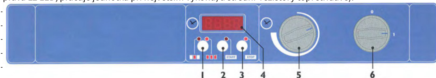
Obr. 1: 1 - hlavní vypínač (jednotky), 2 - tlačítko startu, 3 - tlačítko stop, 4 - tlačítko reset, 5 - regulace teploty, 6 - regulace výkonu
